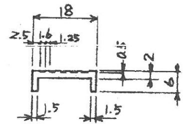
棚枠断面 S=1
