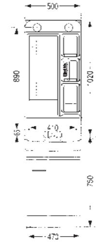
※写真は、T-500S単水栓タイプです。 ※図面は、T-500C 2ハンドル混合水栓付きタイプです。
