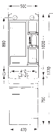
※図面は、T-500C 2ハンドル混合水栓付きタイプです。
